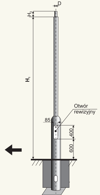
MSO... - 2 dwustopniowe
