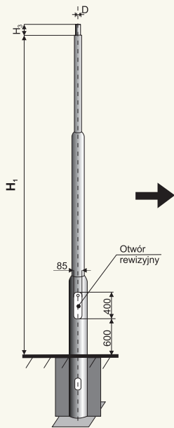
MSO... - 3 trzystopniowe
