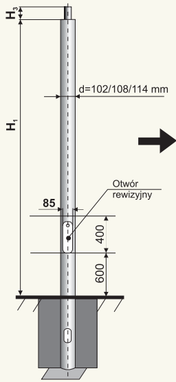
MSO... - 1 jednostopniowe
