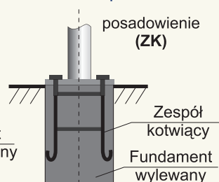
posadowienie (F)
