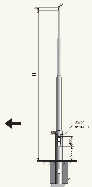
MSO... - 4 czterostopniowe
