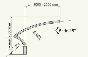
Wysięgnik łukowy łamany WLL
