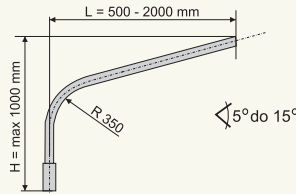
Wysięgnik łukowy mały WŁM
