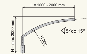
Wysięgnik łukowo - kątowy WŁK
