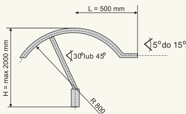
Wysięgnik kątowy - kołowy WKK 1
